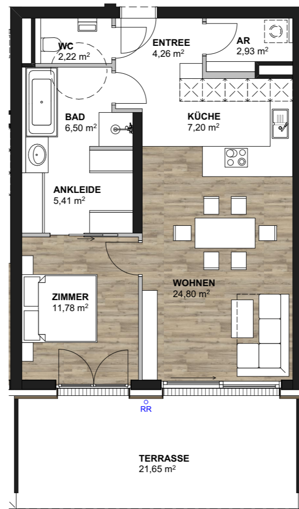
HAUS 1 TOP 2 M 1:100
