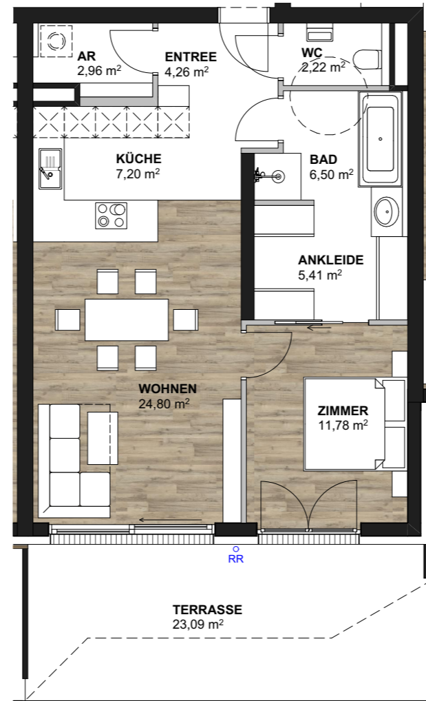
HAUS 1 TOP 3 M 1:100
