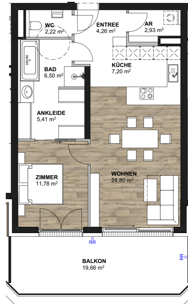
HAUS 1 TOP 6 M 1:100
