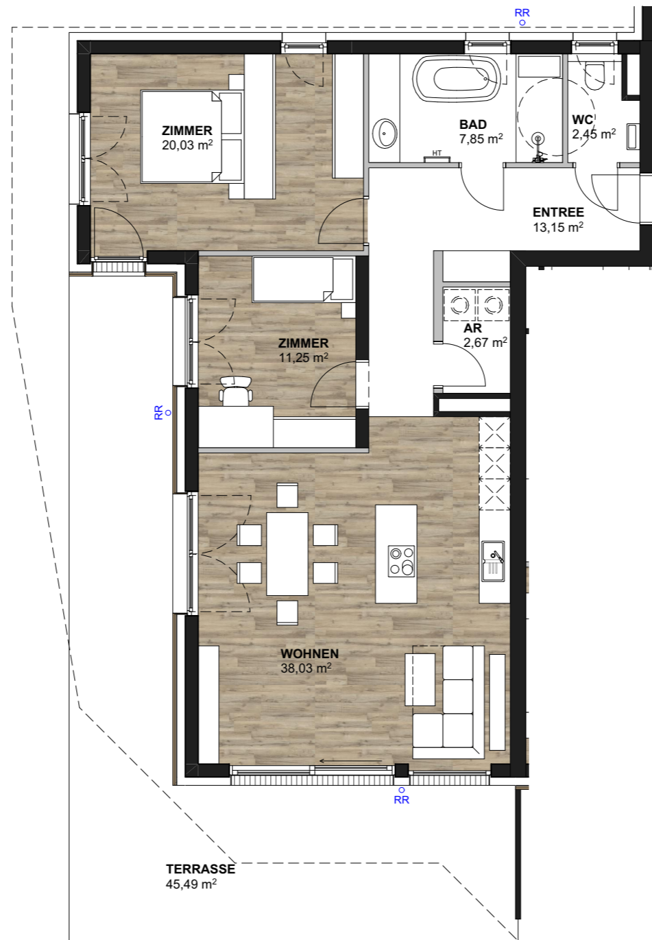
HAUS 2 TOP 1 M 1:100
