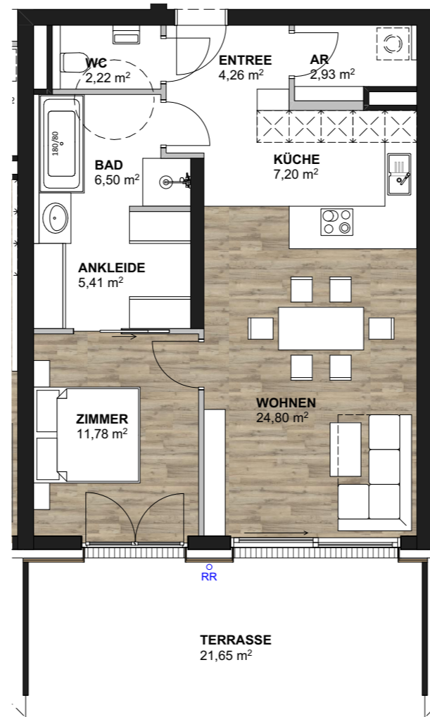
HAUS 2 TOP 2 M 1:100
