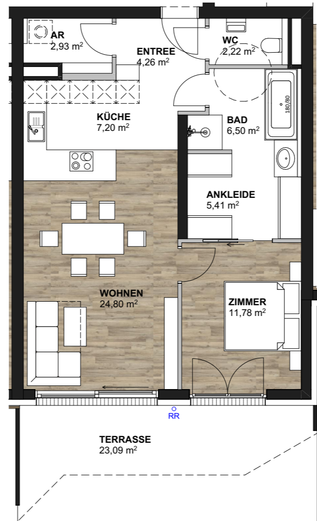
HAUS 2 TOP 3 M 1:100
