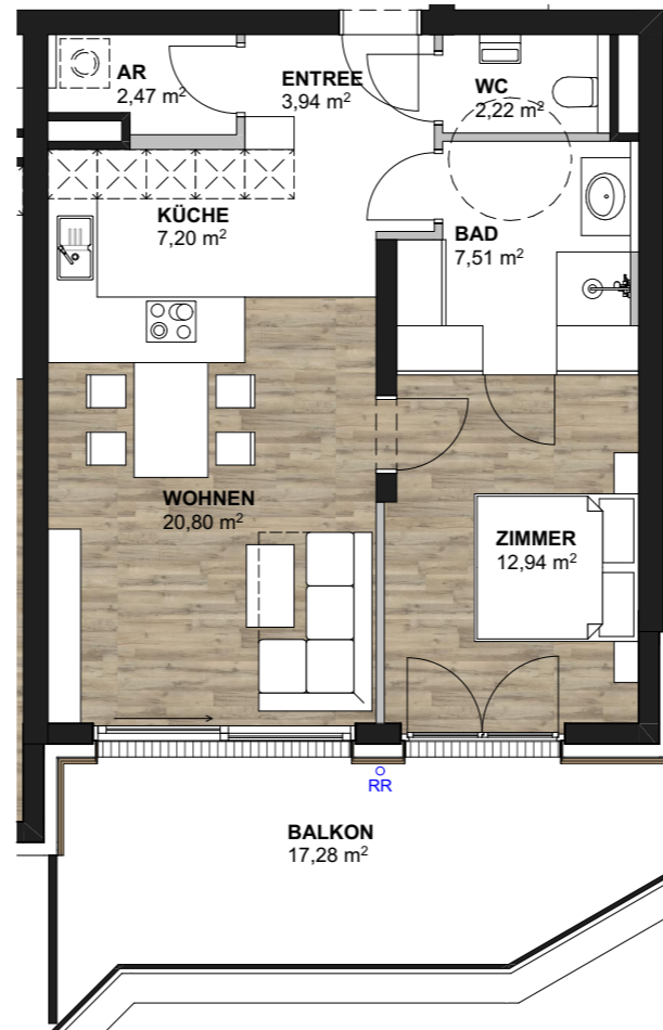
HAUS 2 TOP 7 M 1:100
